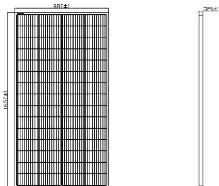
а) Вид спереди б) Вид сбоку Рисунок 1 – Схематическое изображение ФЭМ.
